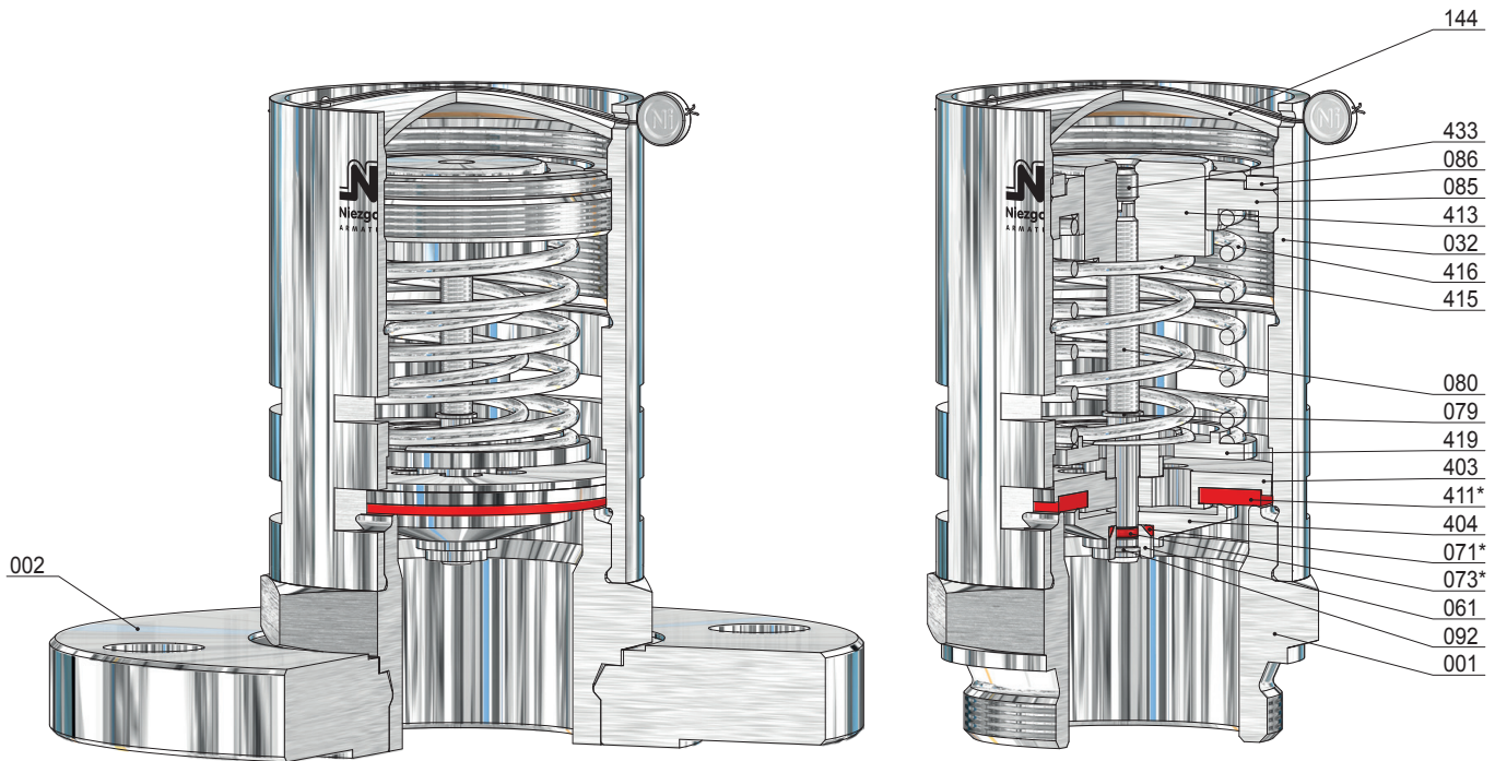
BG III mit Flanschanschluss nach z.B. DIN / ASME
