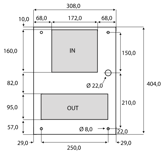
Montageausschnitt bei Aufbaumontage
